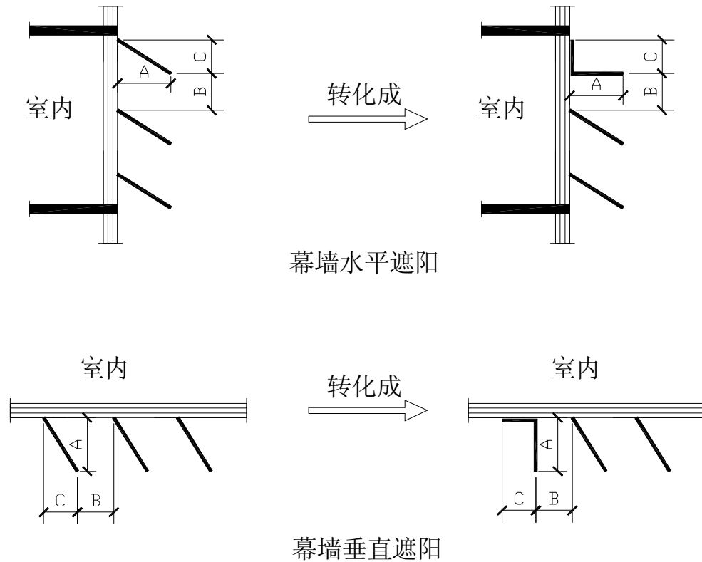
图 A.0.4 幕墙遮阳计算示意
